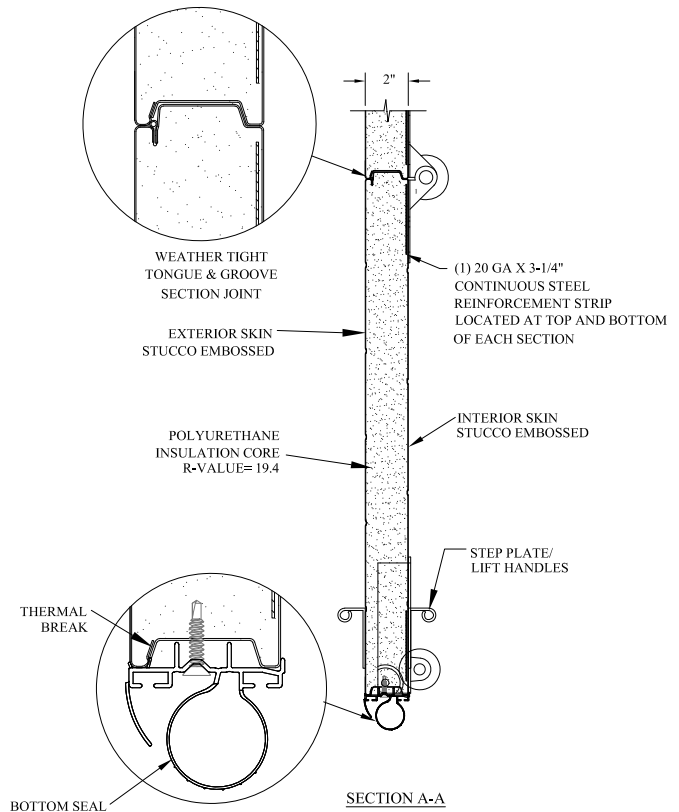
SECTION A-A
